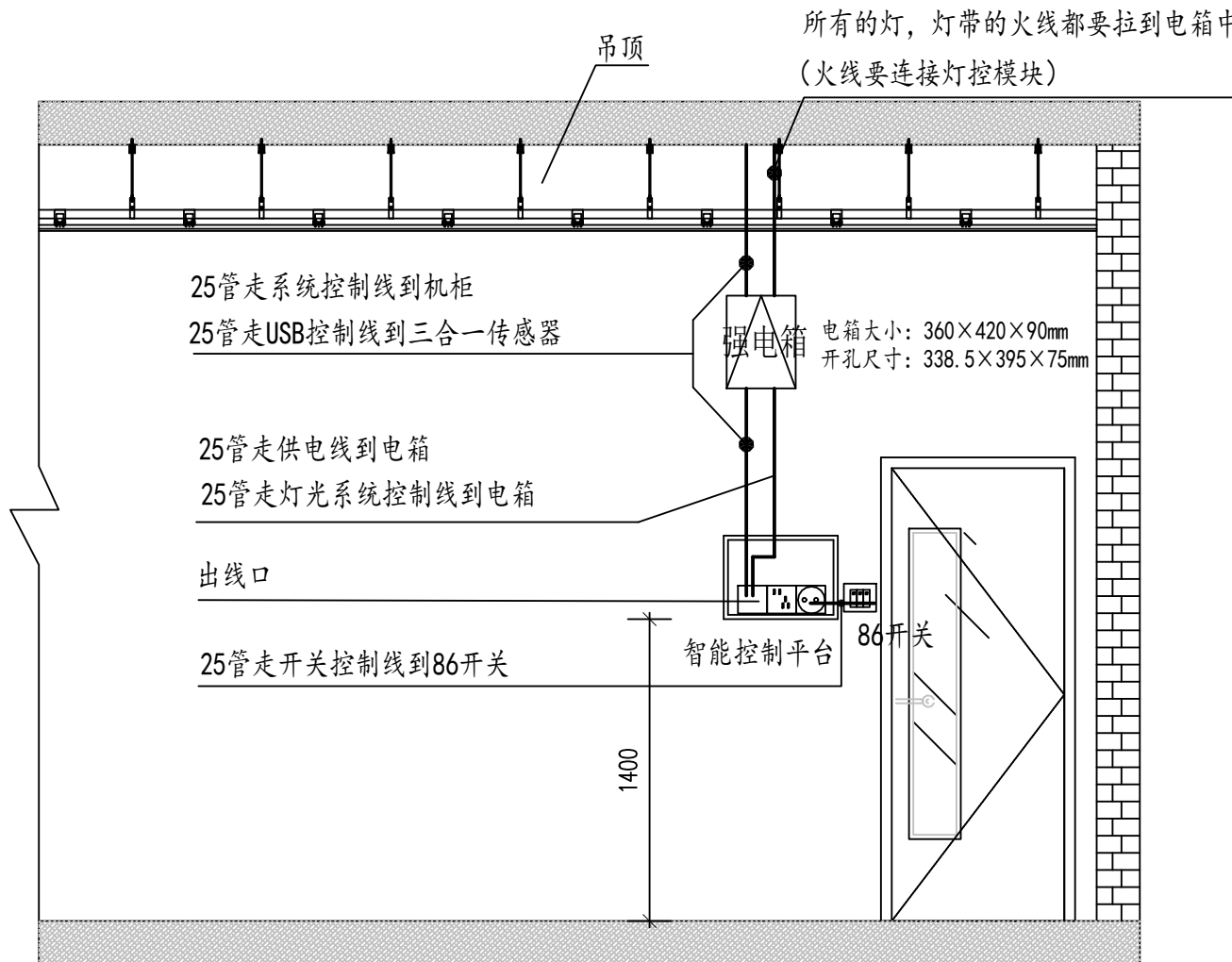
重庆市中医骨科医院一体化智能阅片会诊中心B面示意图2(放大图)
