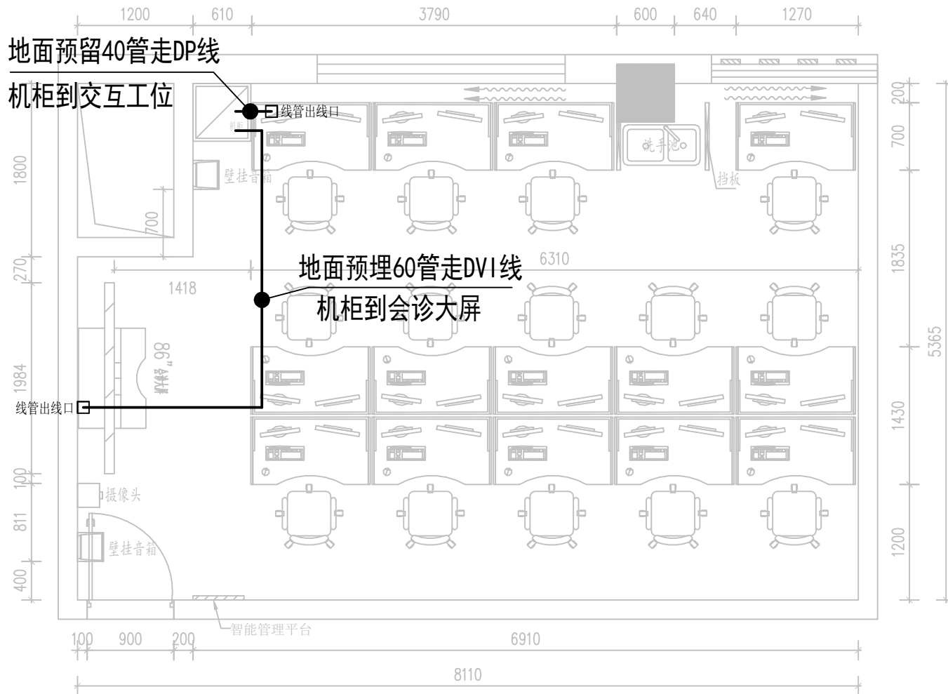
重庆市中医骨科医院一体化智能阅片会诊中心地面走线图
