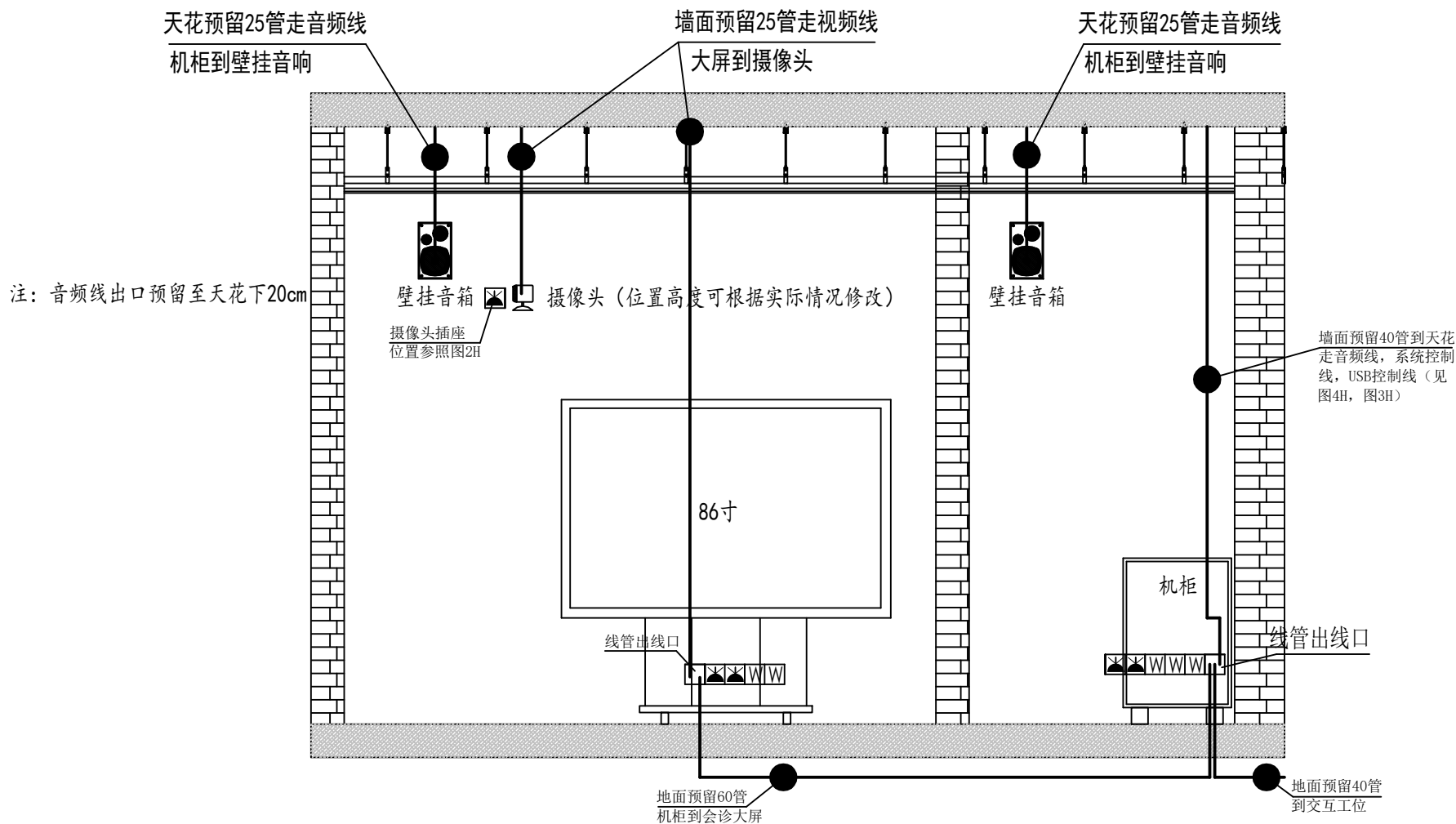
重庆市中医骨科医院一体化智能阅片会诊中心C面示意图2(放大图)
