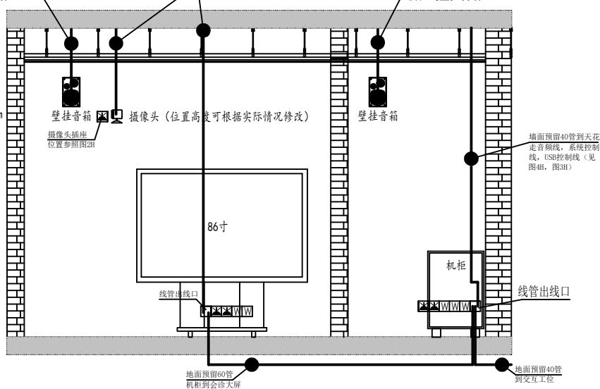
重庆市中医骨科医院一体化智能阅片会诊中心C面示意图1
