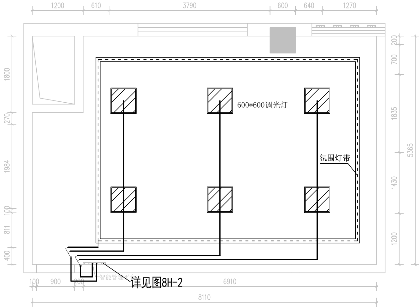
重庆市中医骨科医院一体化智能阅片会诊中心灯光控制图
