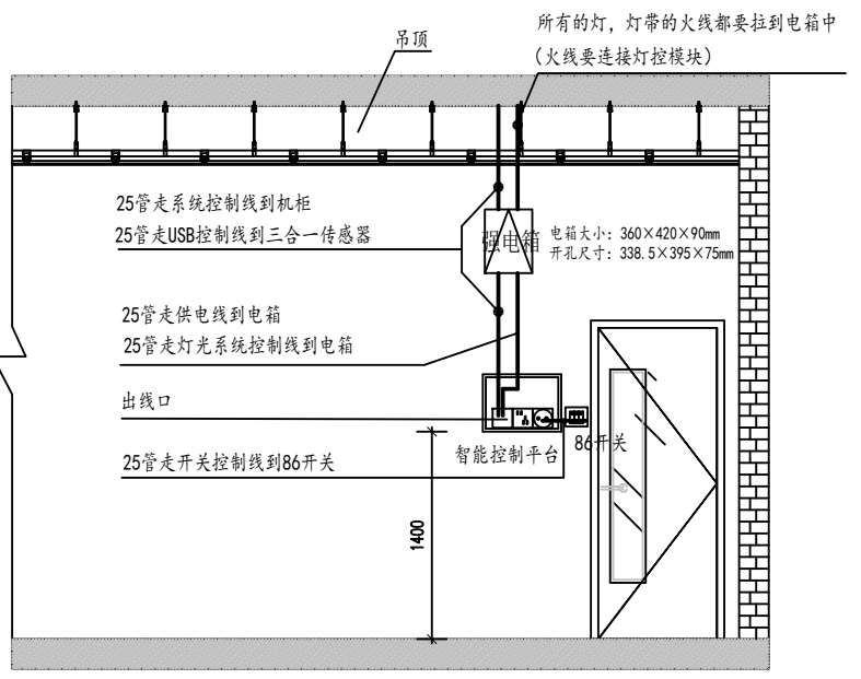
重庆市中医骨科医院一体化智能阅片会诊中心B面示意图1
