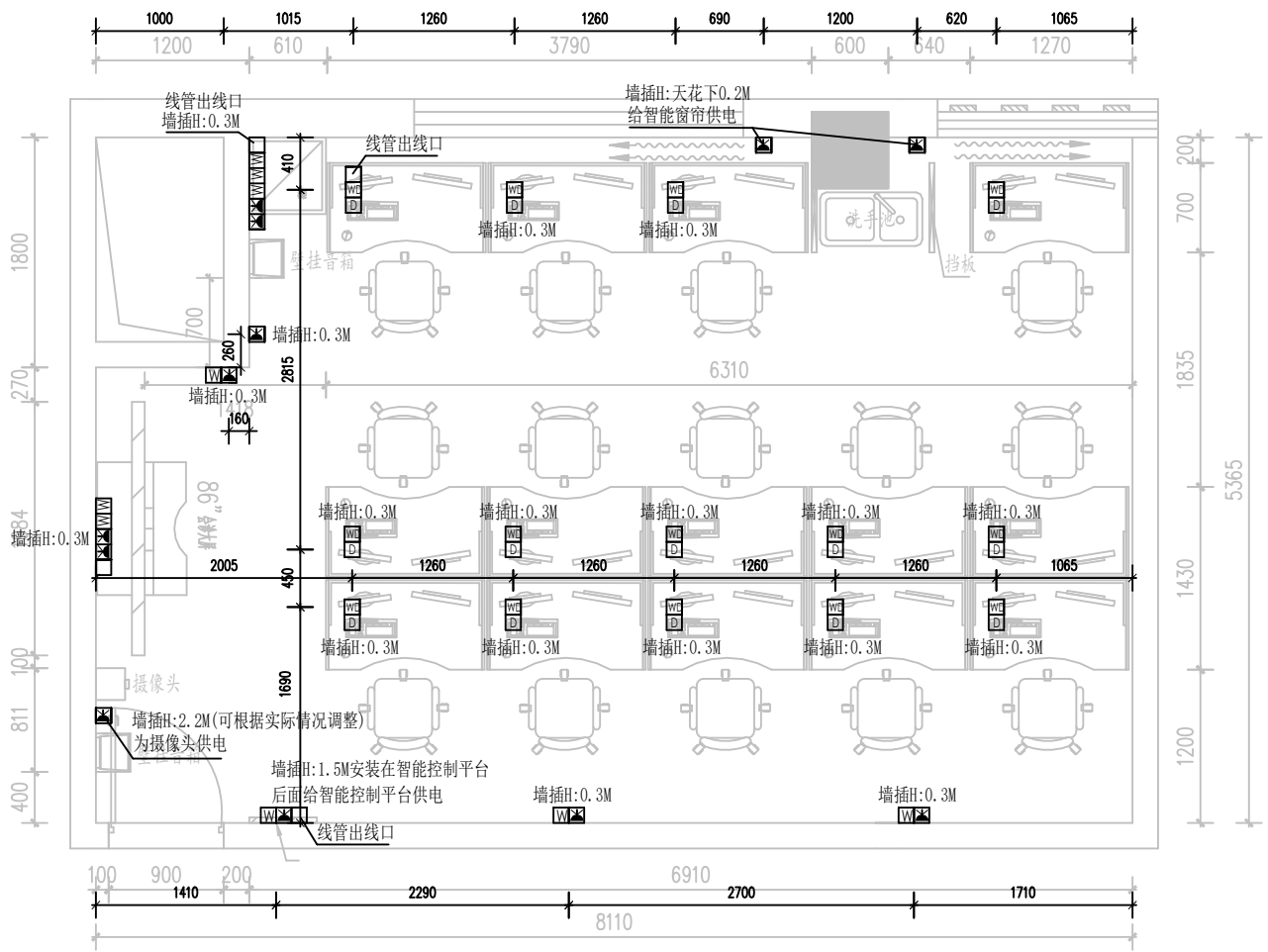
重庆市中医骨科医院一体化智能阅片会诊中心插座点位图
